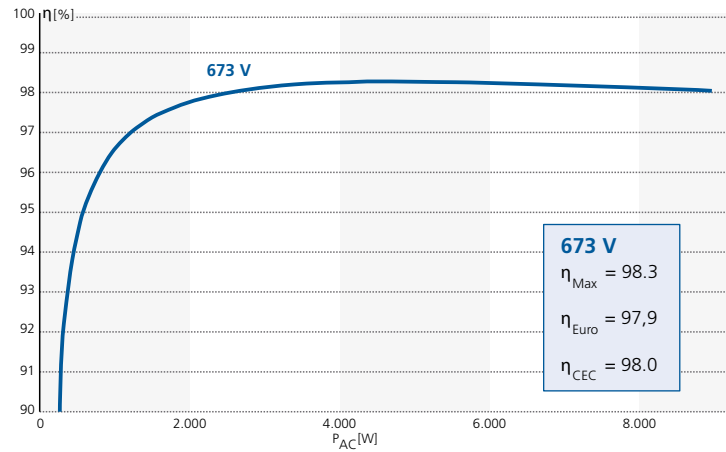
Wirkungsgradkennlinie blueplanet 9.0 TL3
